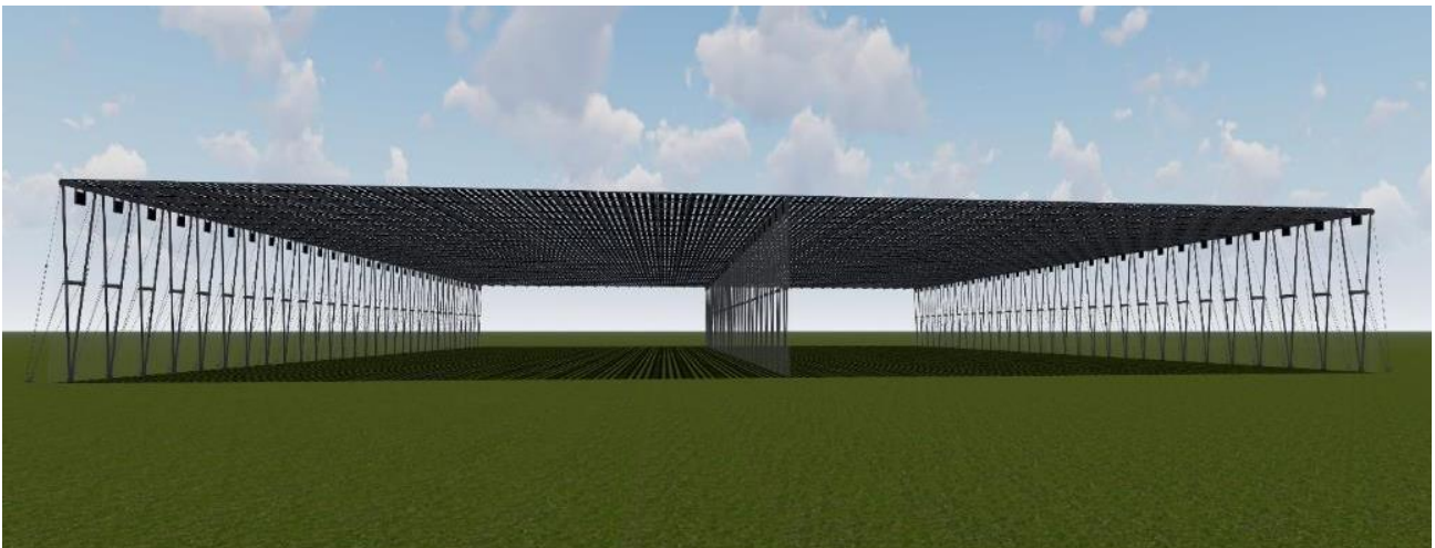
MABEWO TerraFlex: Die leichte Konstruktion ist mit vielen technischen Optionen ausrüstbar: transparenten Paneelen, Folien, Bewässerung, Sensortechnik u.v.m.
